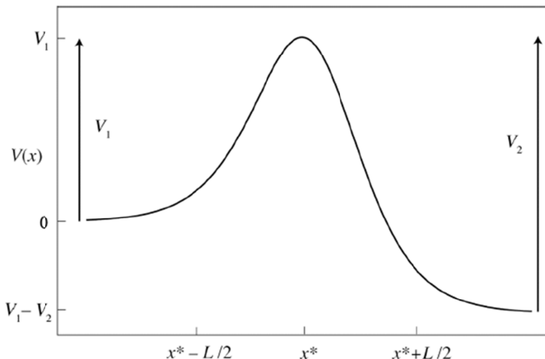
5. ábra Az Eckart-potenciál sematikus ábrázolása
