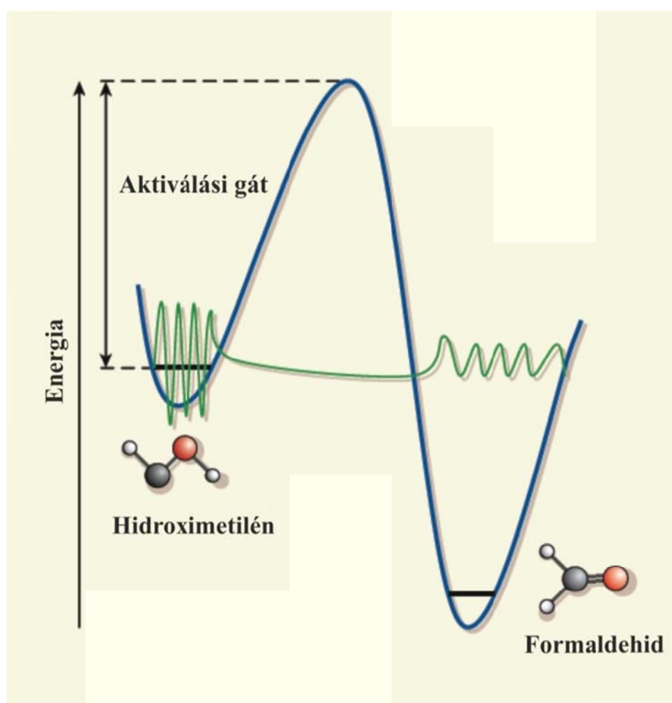
4. ábra A trans -HCOH → H 2 CO izomerizációs reakció 1,2-H-eltolódás mechanizmusú alagúthatással történő lejátszódása.
